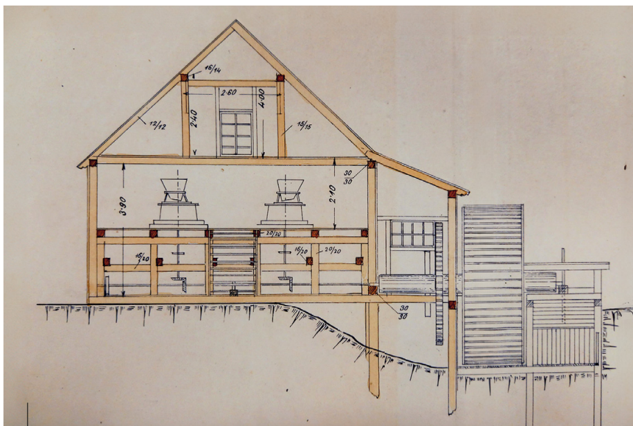
Projekt młyna na Kobylakach Antoniego Teleckiego z roku 1926
